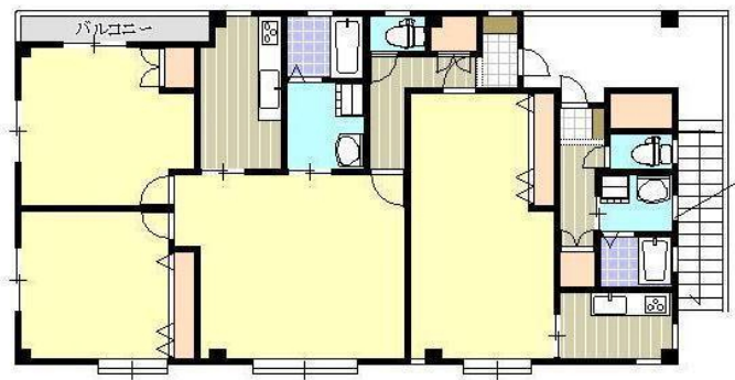
2階平面図(約35坪)
