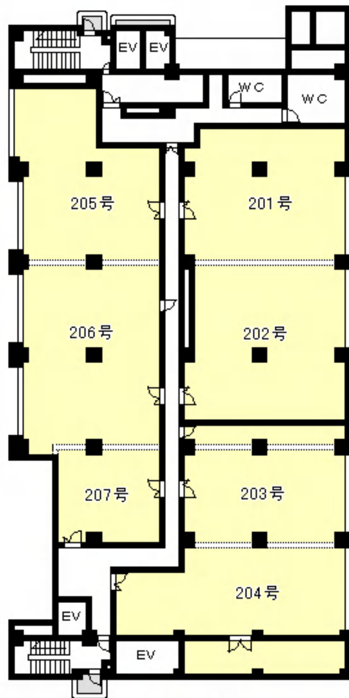
2階 平面図
